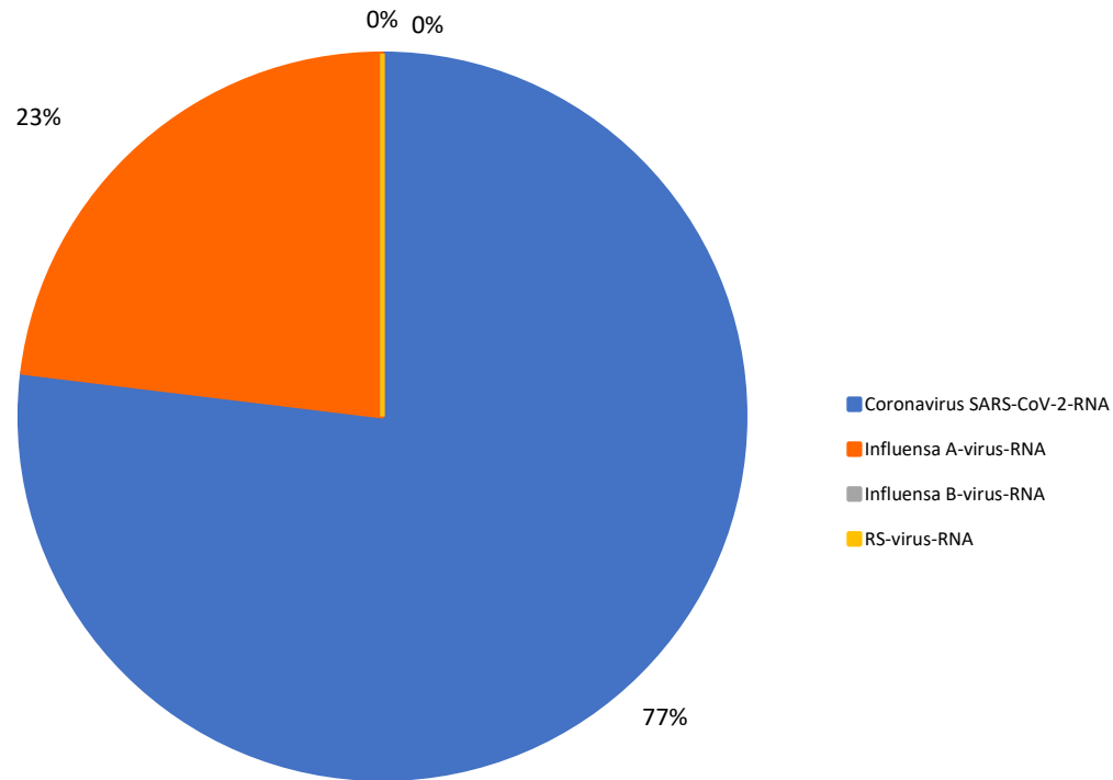
Beställning Corona SARS-CoV-2/Influensa/RSV, Akut (GeneXpert) andel positiva fynd = 4 %, antal testade prov = 312
