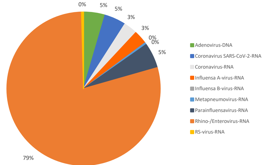
Beställning Luftvägspanel (QiaStat) andel positiva fynd = 36 %, antal testade prov = 777
